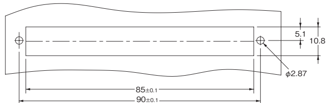
面板加工尺寸 (顶视图)
