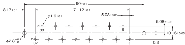
印刷电路板加工尺寸 (底视图)
