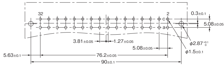
面板加工尺寸 (顶视图)
