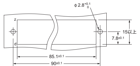
面板加工尺寸 (顶视图)
