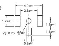
印刷基板焊盘尺寸示例 (TOP VIEW)
