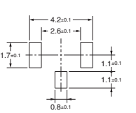
印刷基板焊盘尺寸示例 (TOP VIEW)
