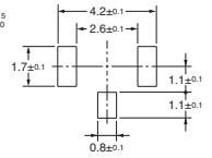
印刷基板焊盘尺寸示例 (TOP VIEW)
