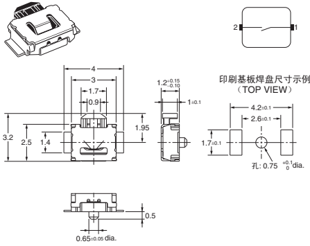
端子配置/内部接线图
