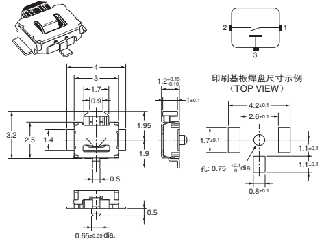
端子配置/内部接线图
